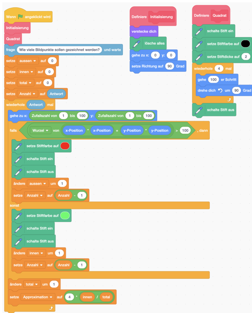
Abbildung 38: «Scratch»-Programm Monte-Carlo.
