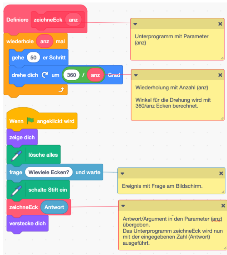
Abbildung 21: Unterprogramm mit Parameter in «Scratch».
