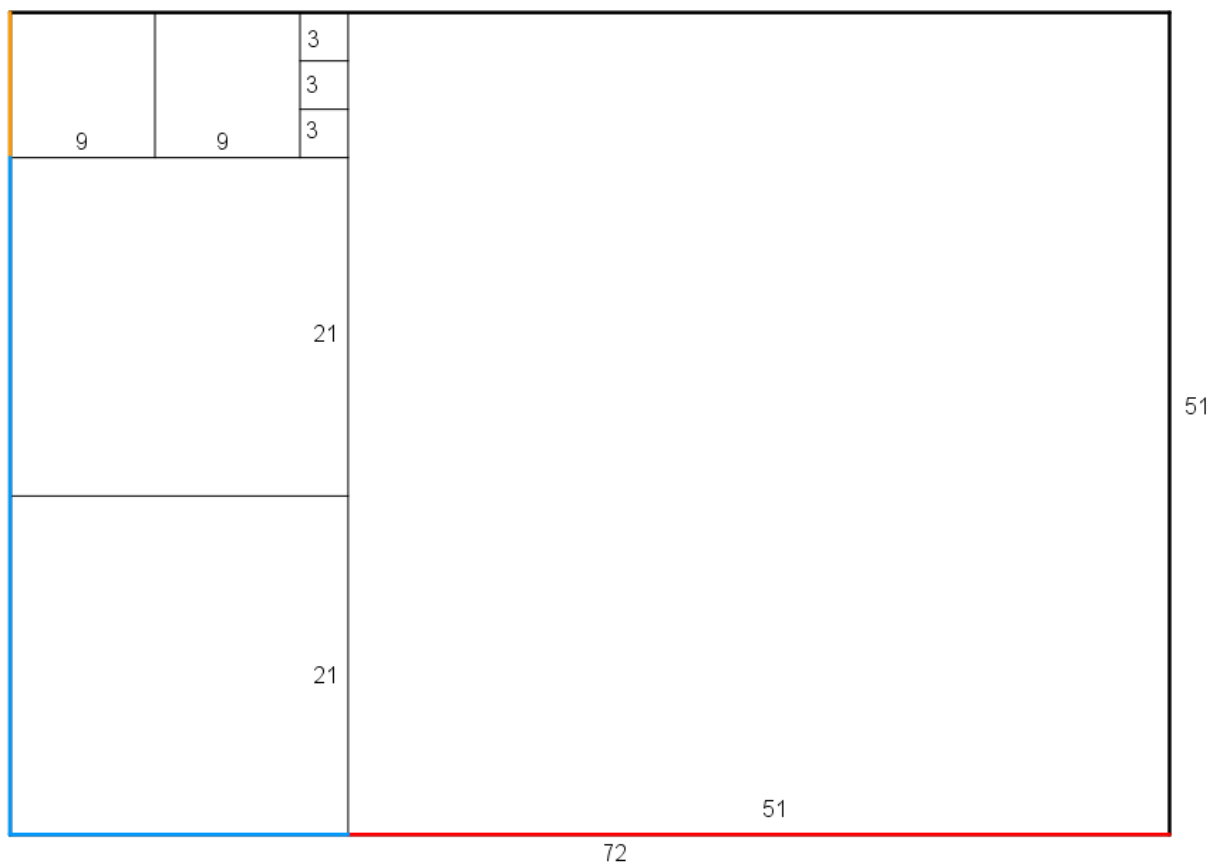
Abbildung 36: Visualisierung des ggT von 72 und 51 mit Hilfe des modernen euklidischen Algorithmus.
