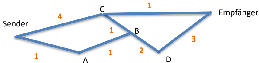
Abbildung 11: Beispiel für eine Aufgabe zum Thema «Routing im Internet», wie sie in Aufgabensammlungen (z.B. im «Informatik-Biber», informatik-biber.ch ) vorkommen: Datenpakete werden vom Sender zum Empfänger geschickt: Welche Route ist die beste, wenn möglichst wenig Kosten (angegeben in grünen Zahlen) verursacht werden sollen? Welche Route ist die beste, wenn über möglichst wenige «Knotenrechner» (A, B, C oder D) gegangen werden soll? (Bettina Waldvogel)
