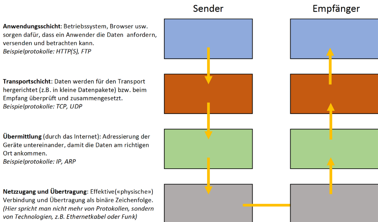
Abbildung 10: Datenversand im Internet. Die vom Sender geschickten Daten durchlaufen den sogenannten «Protokoll-Stack» (Stapel) von oben nach unten: Zwei Protokolle koordinieren Anwendung und Transport (Schicht blau und braun), dann folgen die Protokolle für Versand und Empfang der Datenpakete (grün) und zuunterst eine technische Schicht, bis hinaus zur Datenübertragung via Kabel oder über WIFI. Beim Empfänger durchlaufen die gesendeten Daten den gleichen Protokoll-Stack in umgekehrter Richtung. Von der technisch-physikalischen Schicht bis ganz hinauf zum Empfänger, der seine Daten bekommt, als wären sie nie unterwegs gewesen. (Lorenz Möschler)
